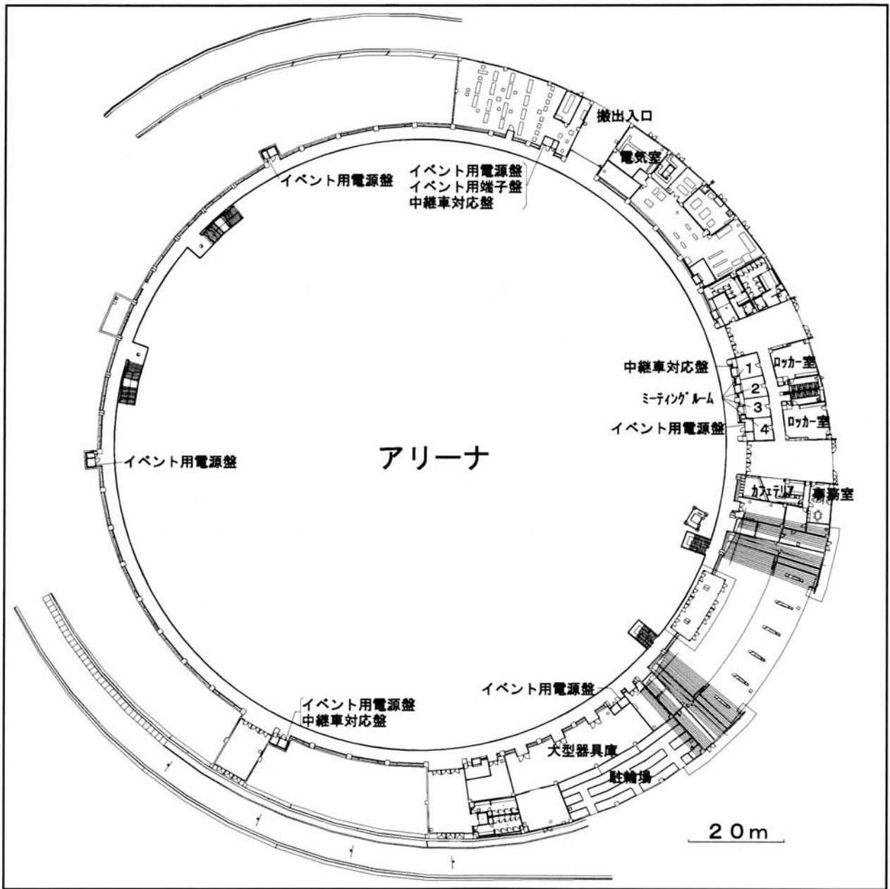
1 階平面図
