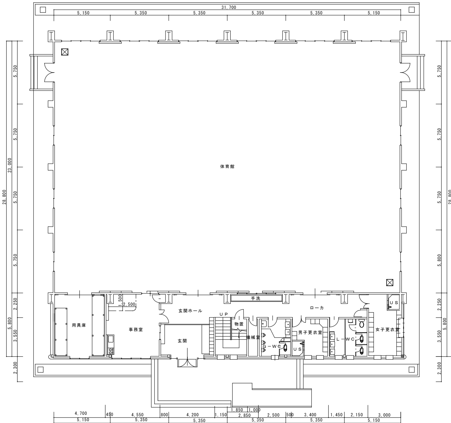
1階平面図
