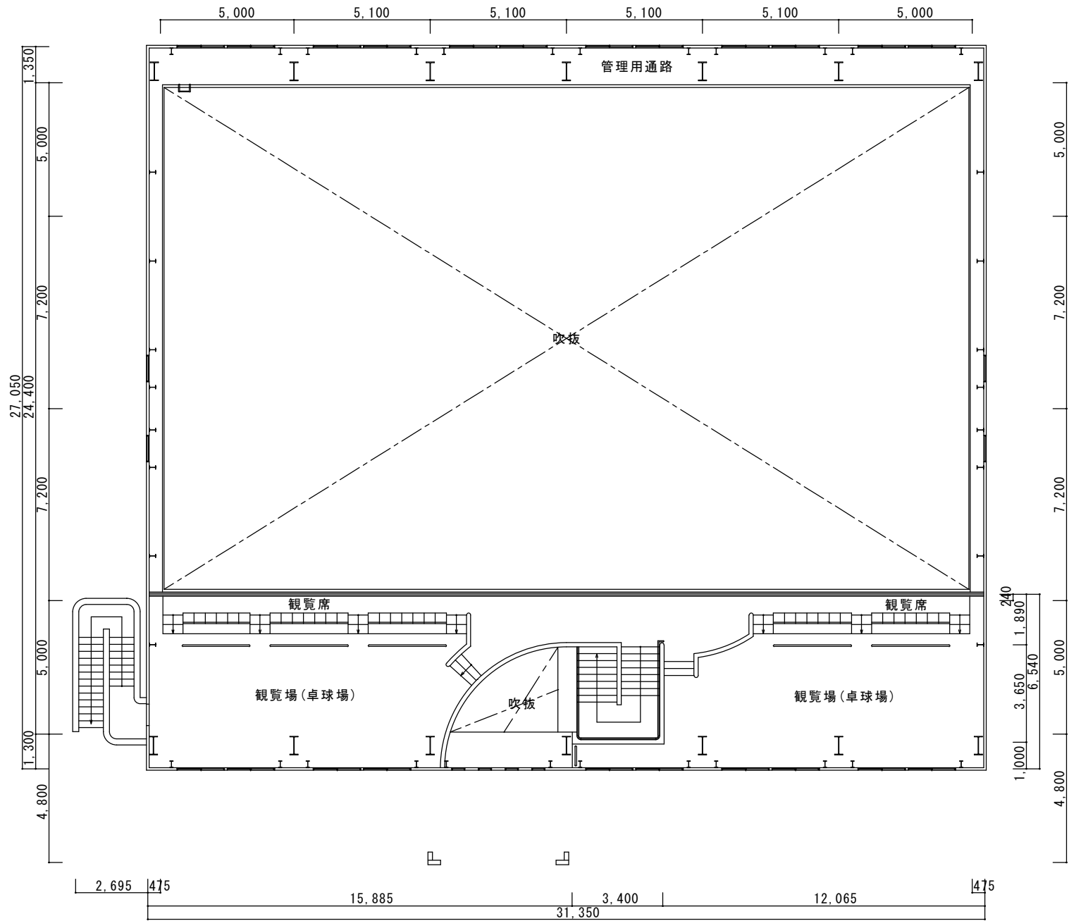
2階平面図 1 : 100
