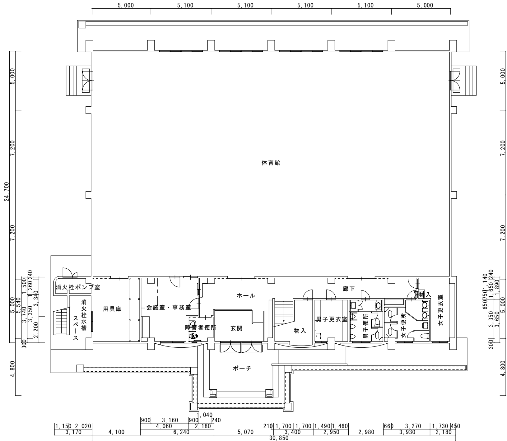
1階平面図 1 : 1 0 0
