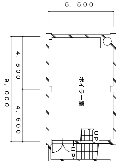
地階平面図 S=1:100
