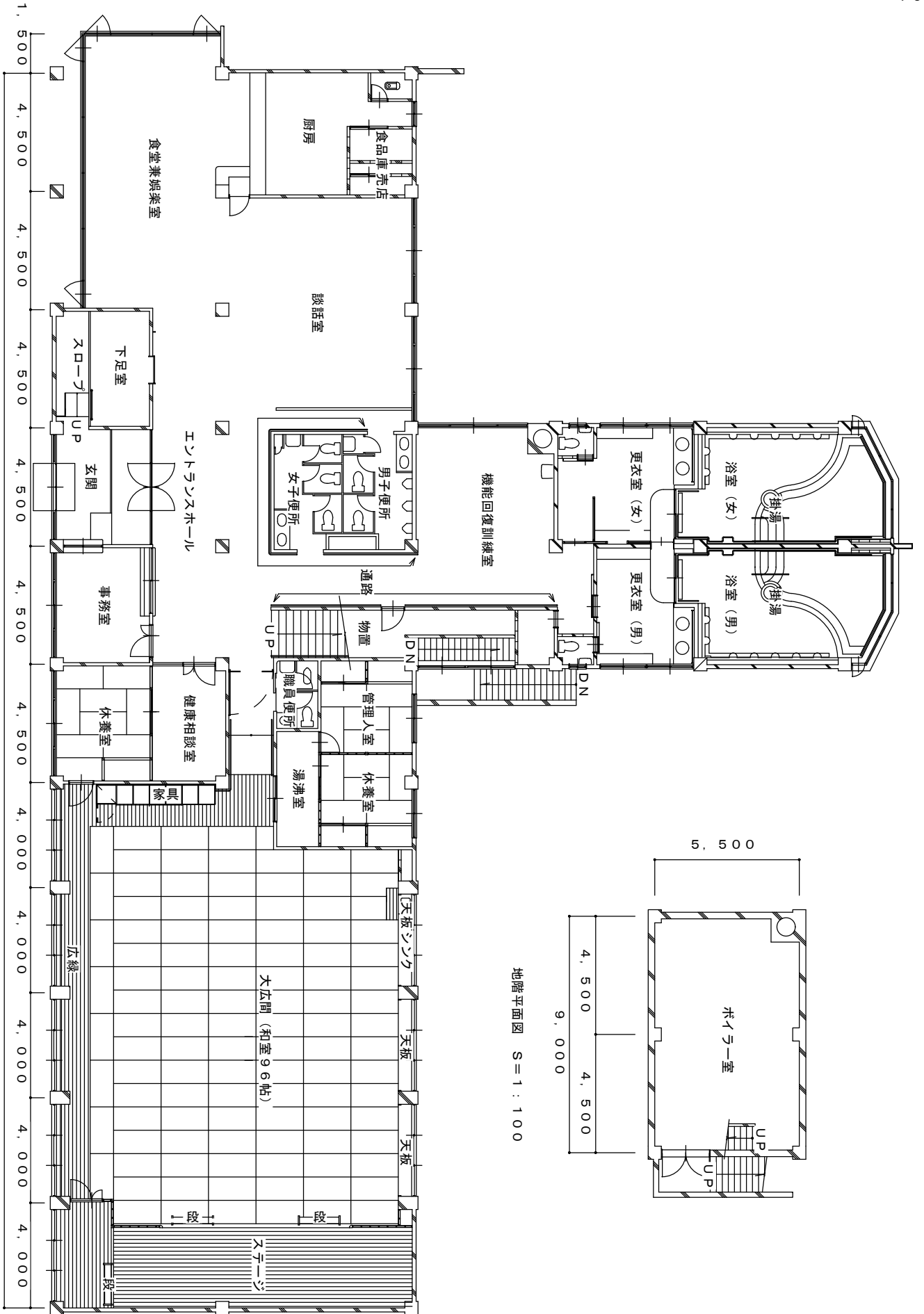
1階平面図 S=1:100
